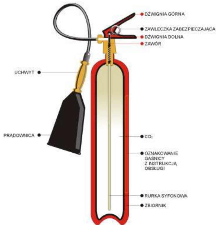
Rysunek 7. Gaśnice śniegowe widok i przekrój
