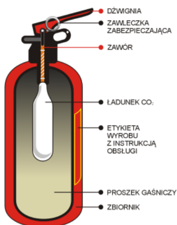
Rys.9 Przekrój gaśnicy typu Z
