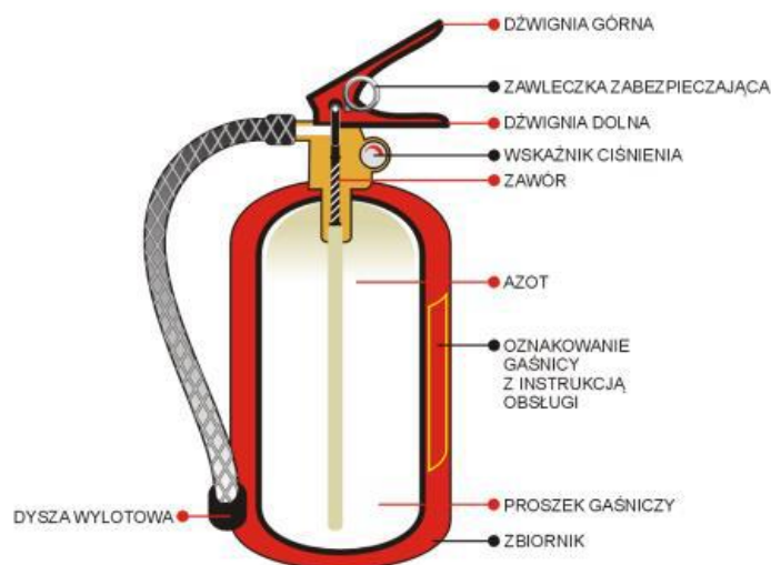
Rys.8 przekrój gaśnicy proszkowej typu X
