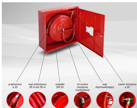
Rysunek 3. Hydrant 25 z węzłem półsztywnym
